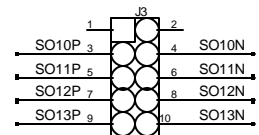
OUTPUT
