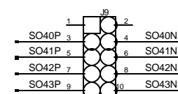
OUTPUT
