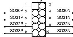
OUTPUT
